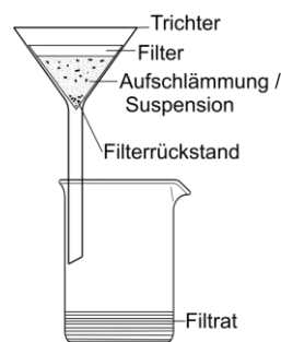
Abb.32: Versuchsaufbau für richtiges Filtrieren im Labor
